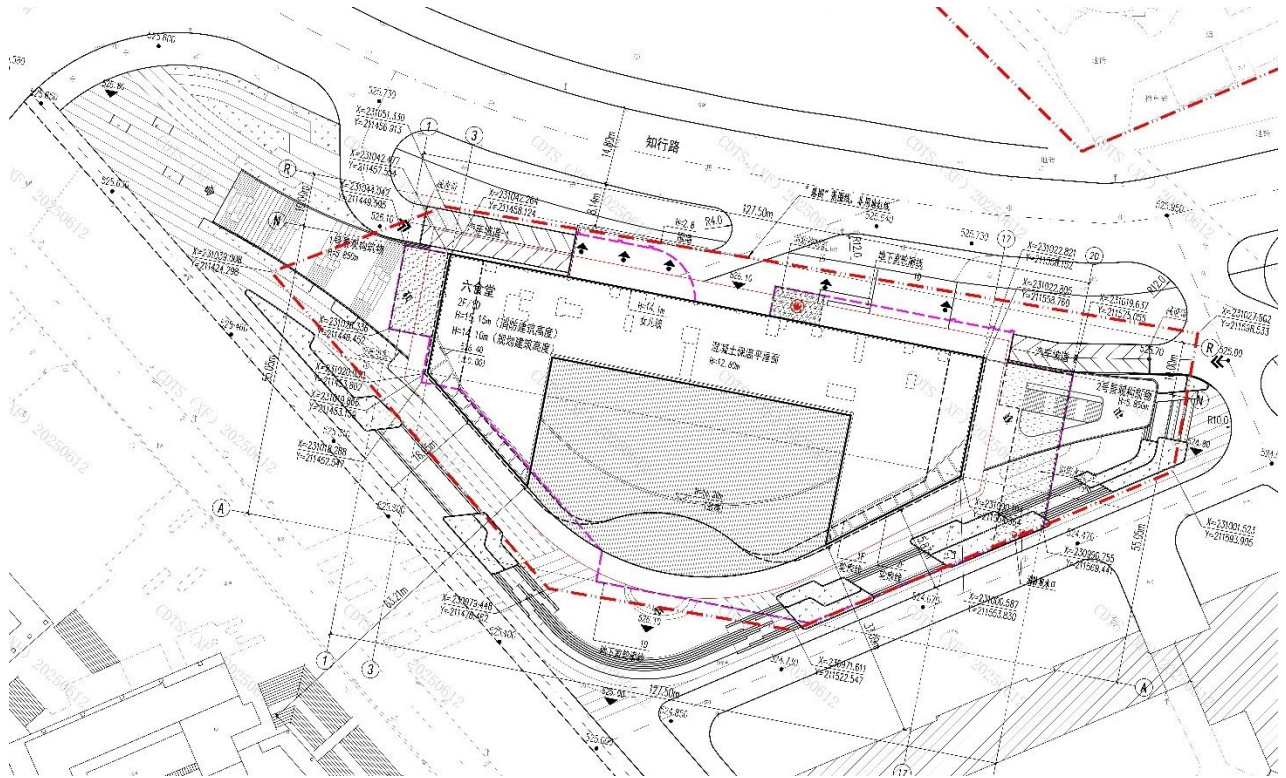
图 1.4-9 项目总平面布置图
