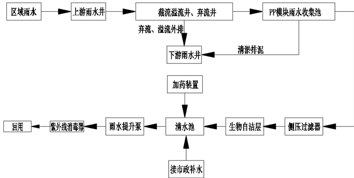
图 1.4-8 雨水处理及回用工艺图
