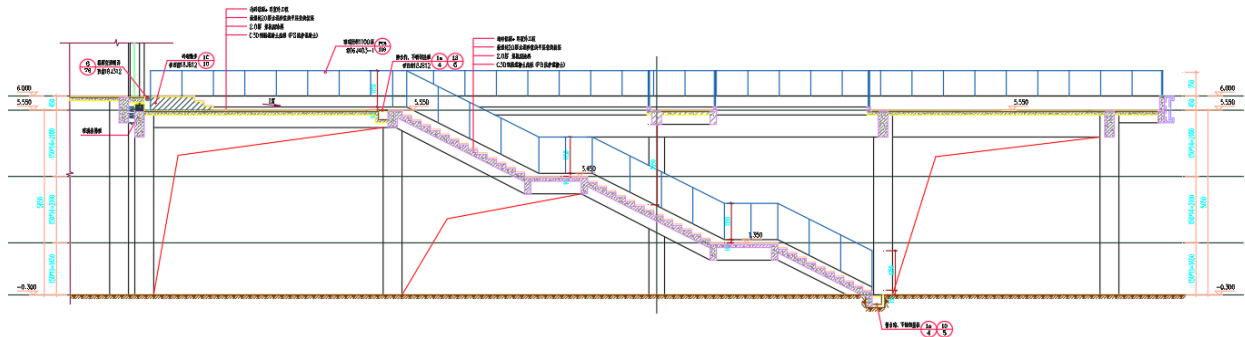
图 1.4-7 2#景观建筑物竖向设计图
